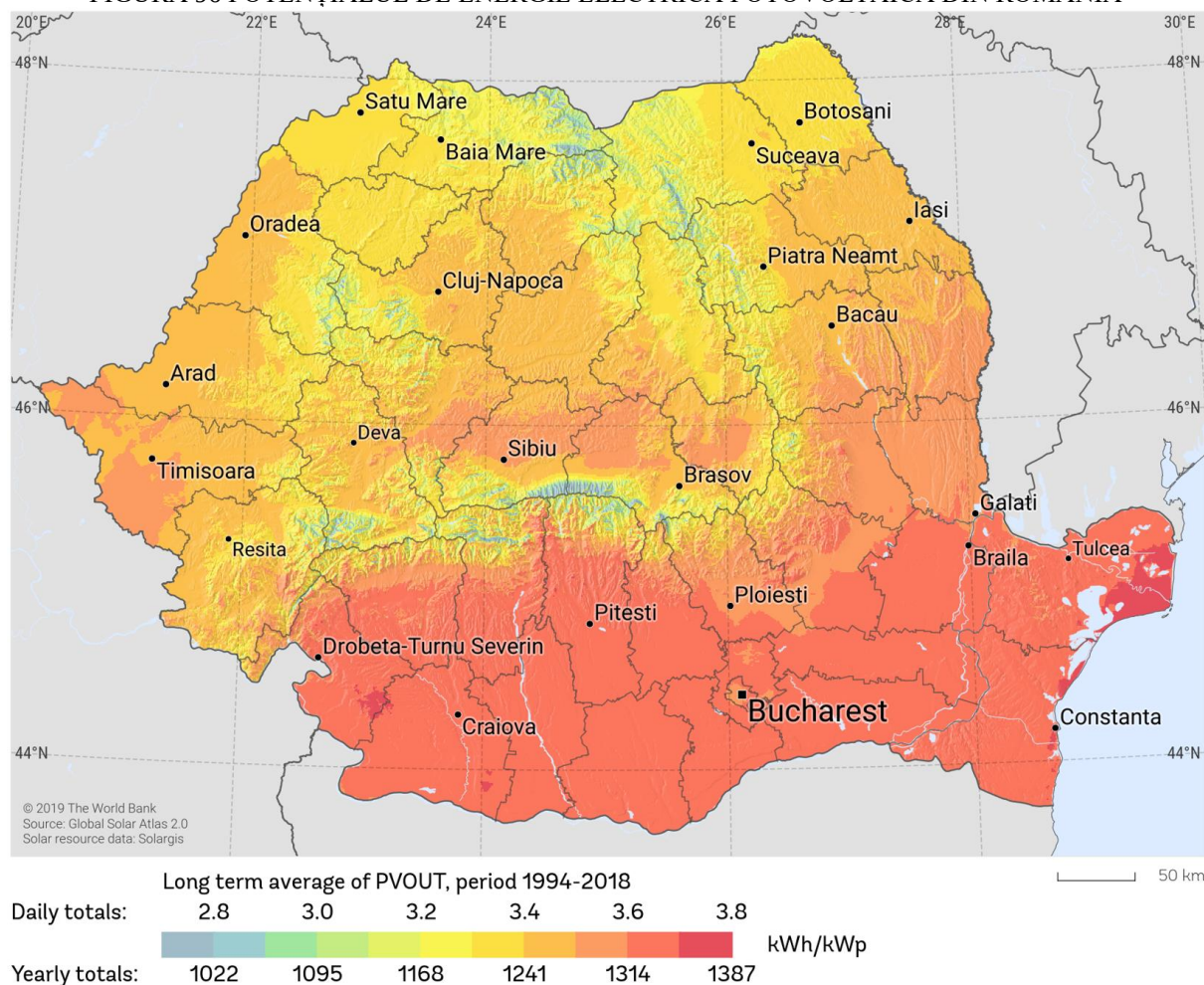
FIGURĂ 96 POTENȚIALUL DE ENERGIE ELECTRICĂ FOTOVOLTAICĂ DIN ROMÂNIA
