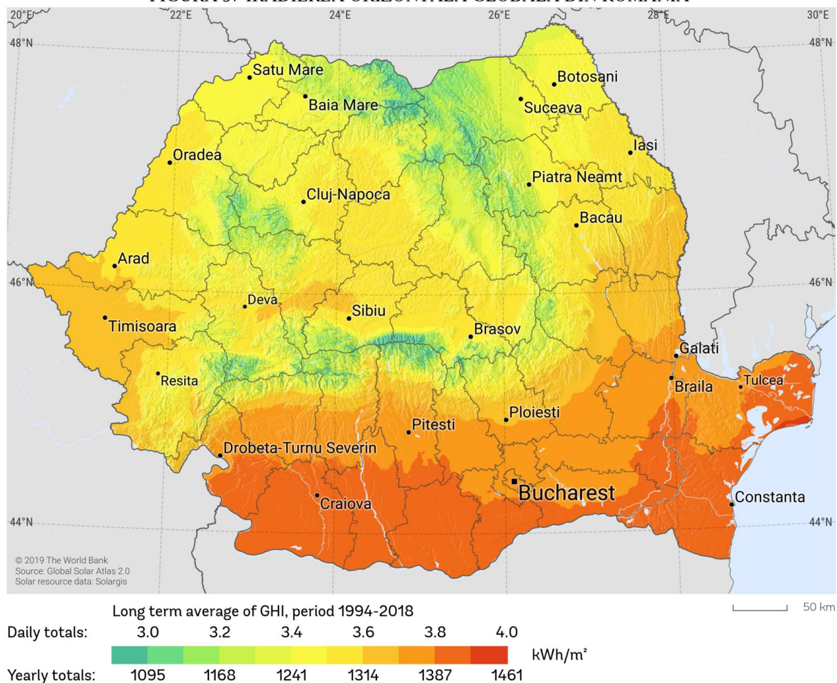
FIGURĂ 97 IRADIEREA ORIZONTALĂ GLOBALĂ DIN ROMÂNIA
